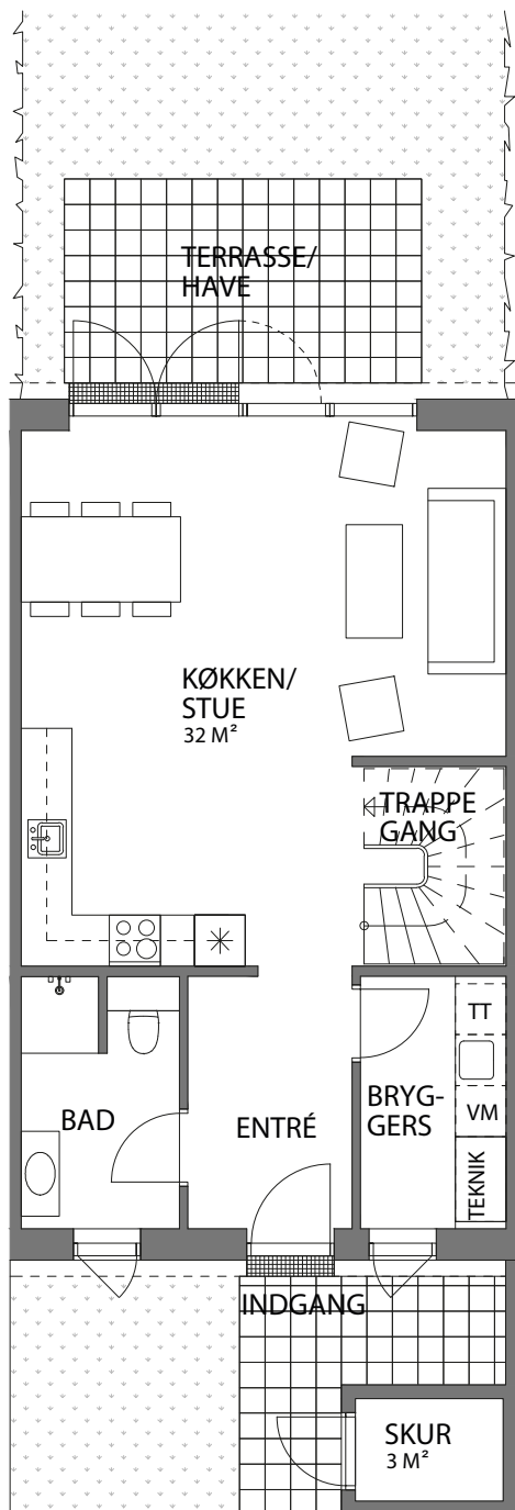
Stueplan
